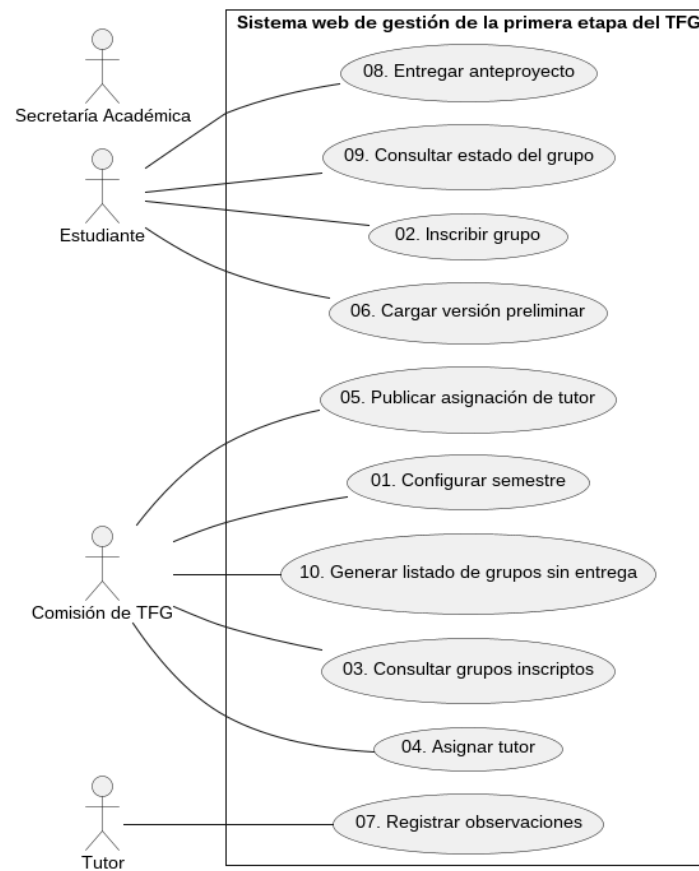
01 — Diagrama general de casos de uso Sistema web de gestión de la primera etapa del TFG
